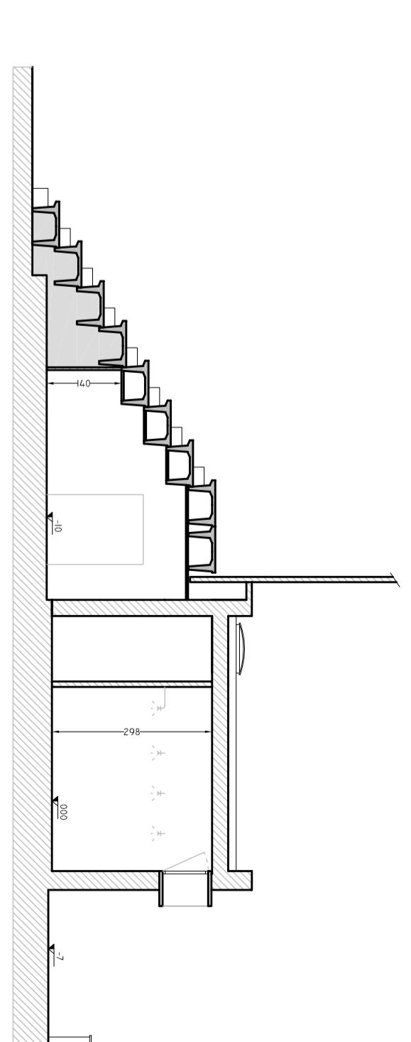
SEZIONE C-C DI RILEVO - SCALA 1:100
