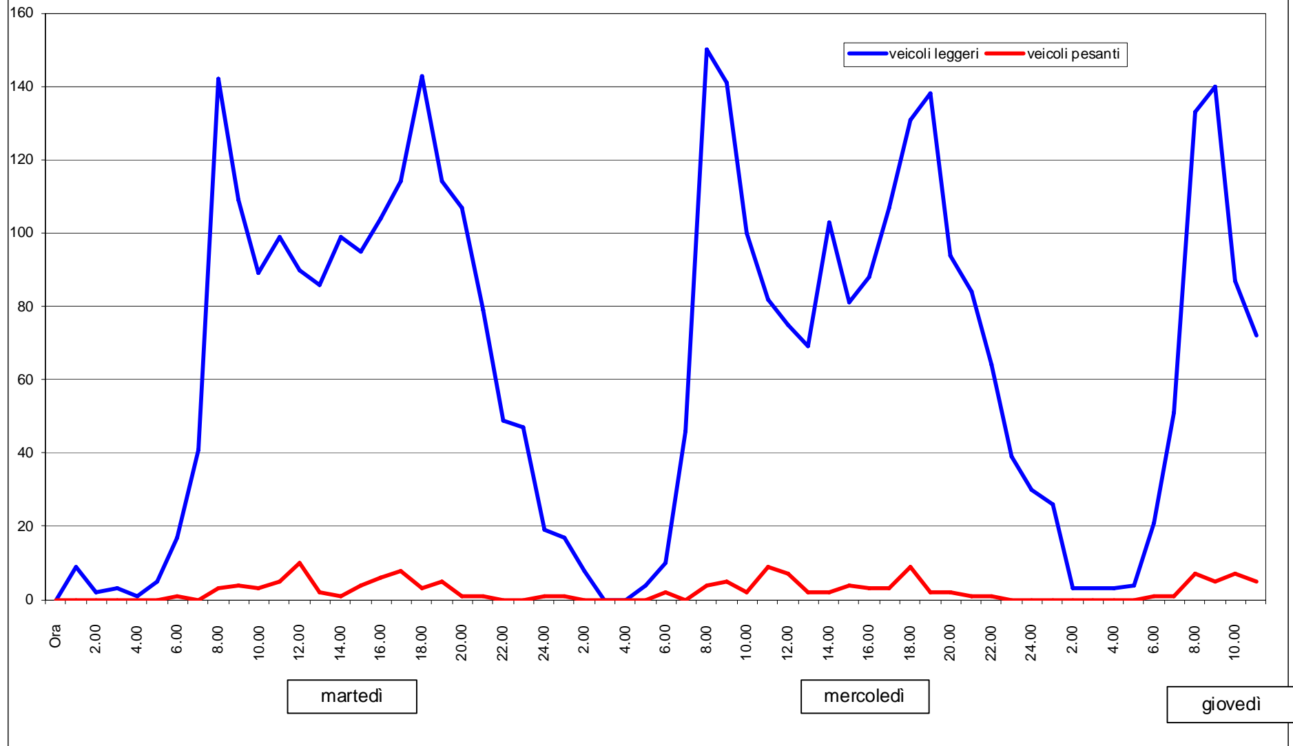
Andamento del traffico da martedì 17 maggio a giovedì 19 maggio 2011 - USCITA
