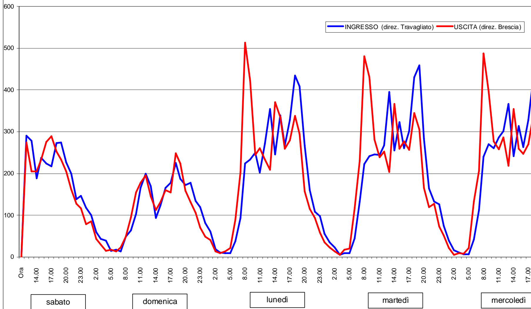
Andamento del traffico da sabato 30 aprile a mercoledì 4 maggio 2011 [veicoli equivalenti]
