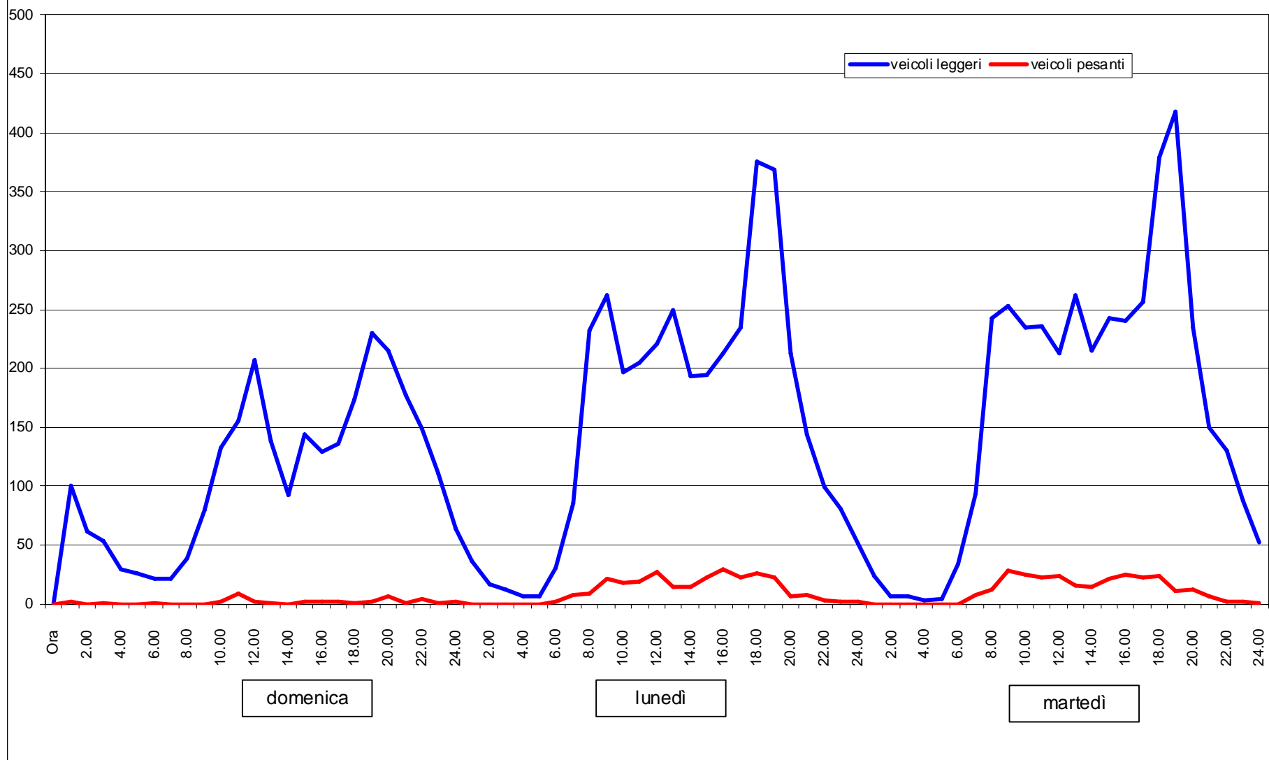
Andamento del traffico da domenica 8 maggio a martedì 10 maggio 2011 - INGRESSO
