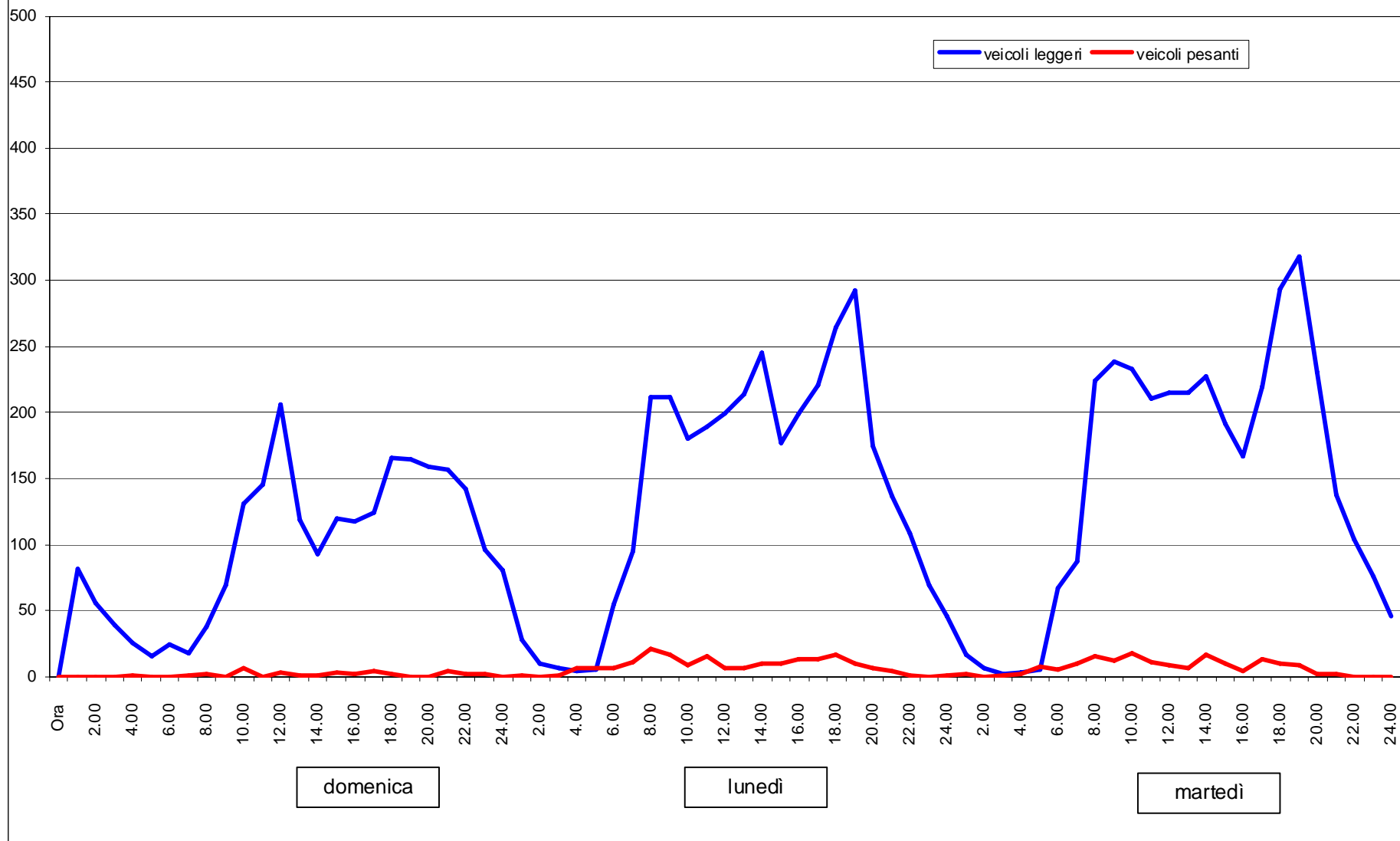
Andamento del traffico da domenica 8 maggio a martedì 10 maggio 2011 - USCITA
