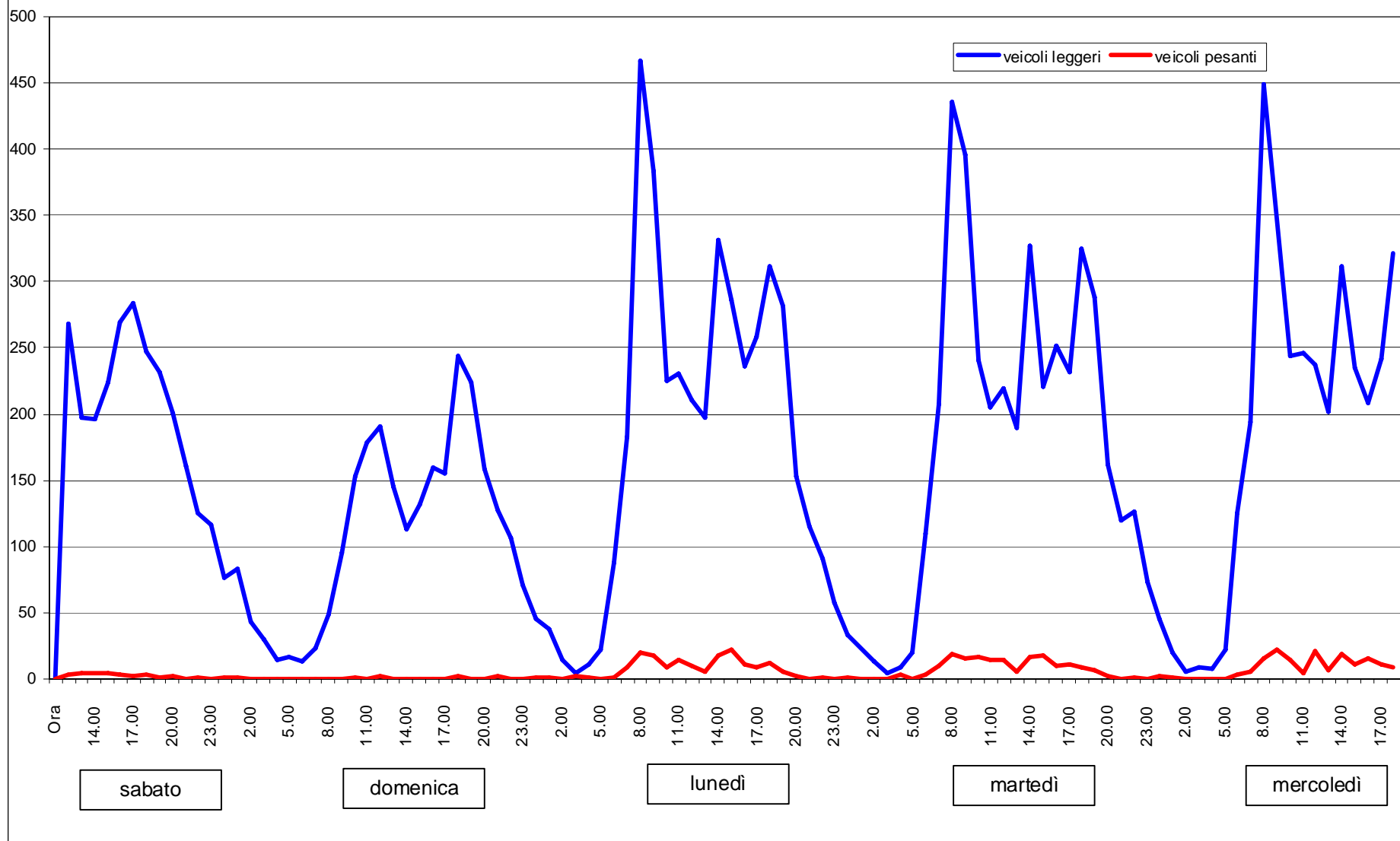
Andamento del traffico da sabato 30 aprile a mercoledì 4 maggio 2011 - USCITA
