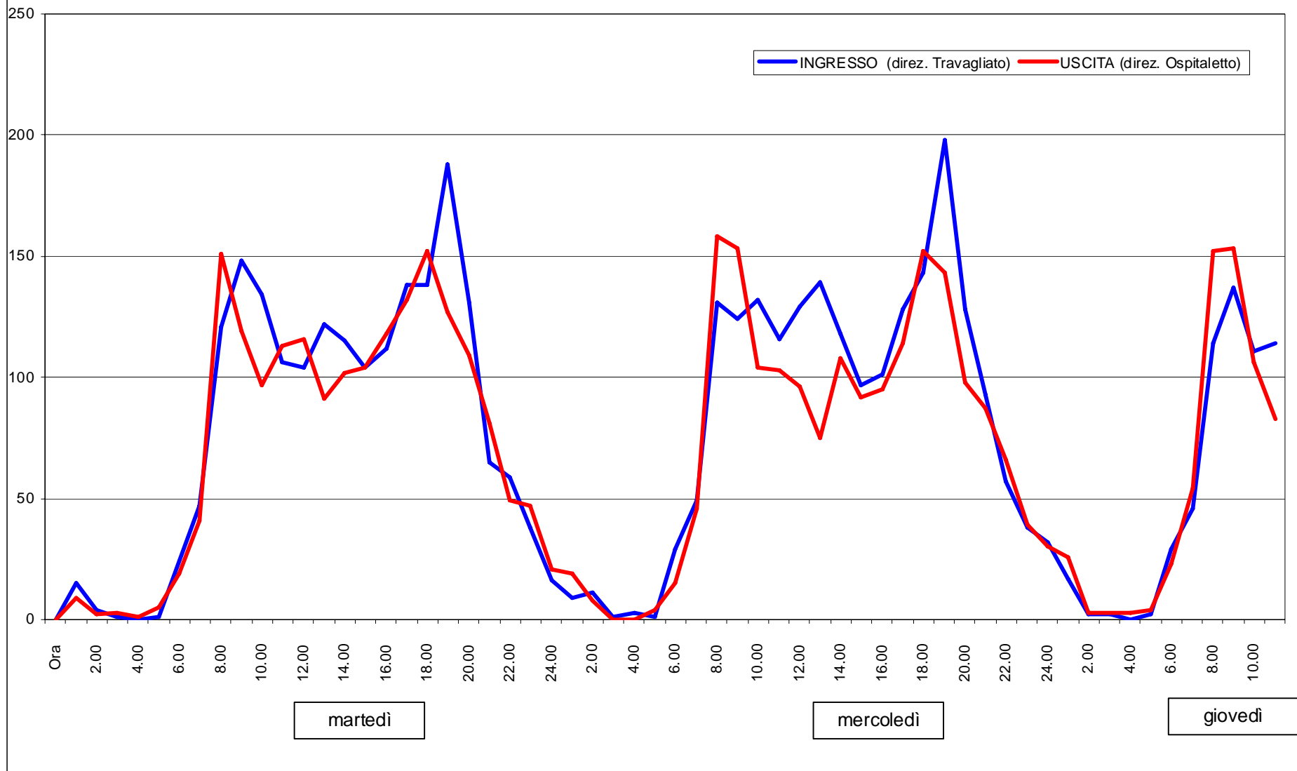
Andamento del traffico da martedì 17 maggio a giovedì 19 maggio 2011 [veicoli equivalenti]
