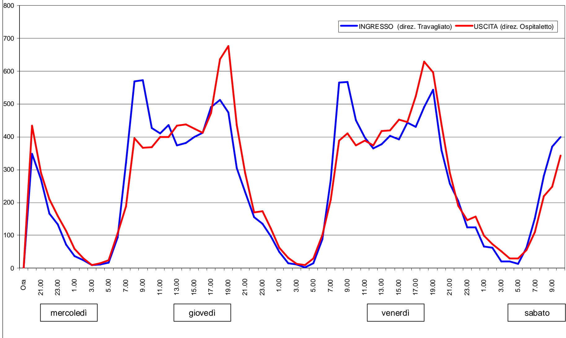
Andamento del traffico da mercoledì 4 maggio a sabato 7 maggio 2011 [veicoli equivalenti]
