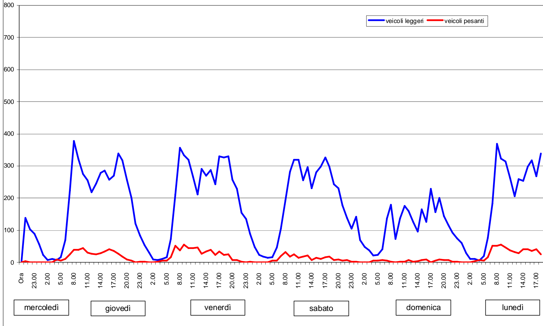
Andamento del traffico da mercoledì 11 maggio a lunedì 16 maggio 2011 - USCITA
