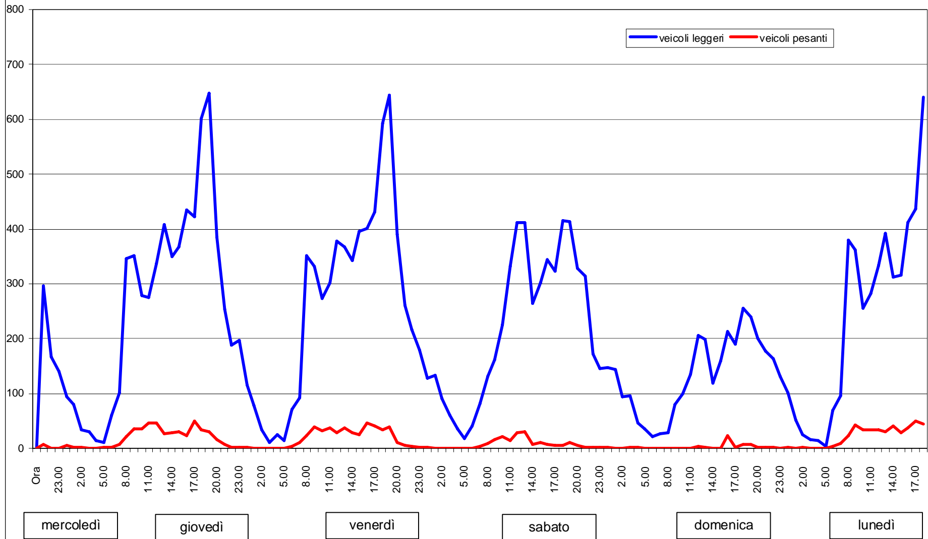
Andamento del traffico da mercoledì 11 maggio a lunedì 16 maggio 2011 - INGRESSO
