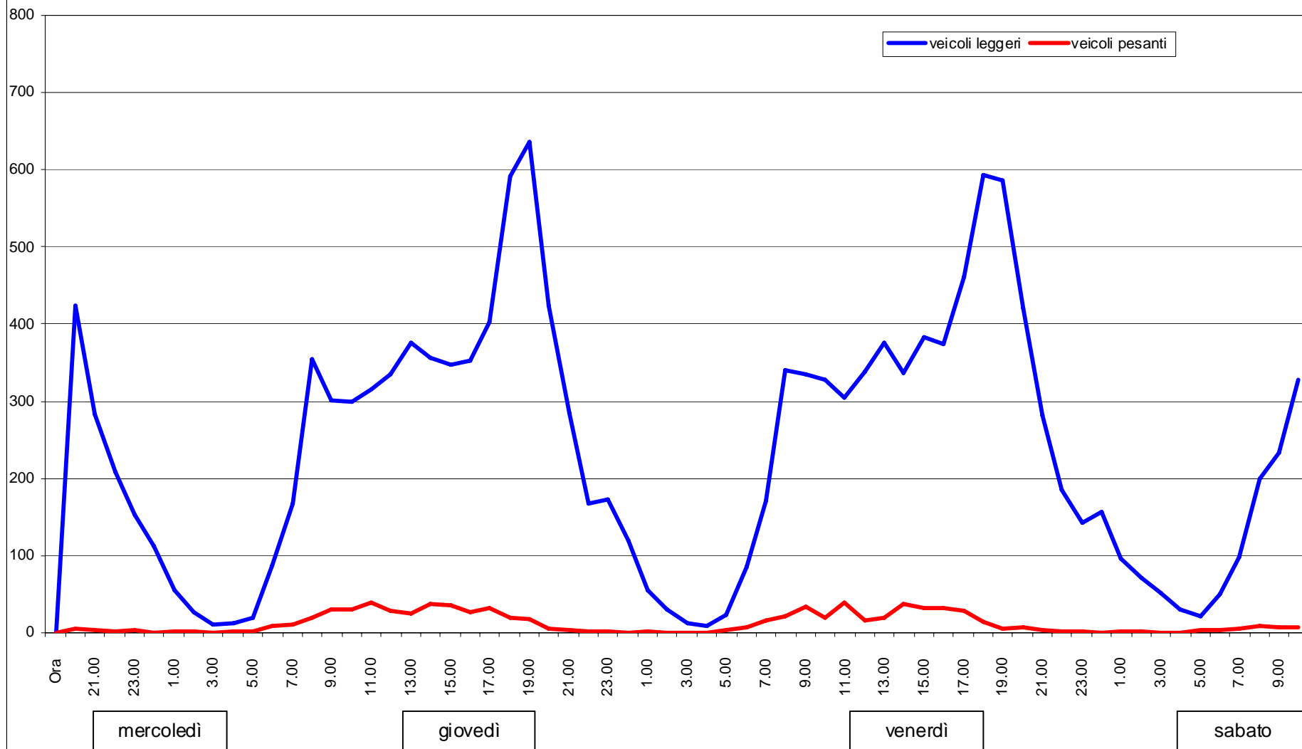
Andamento del traffico da mercoledì 4 maggio a sabato 7 maggio 2011 - USCITA
