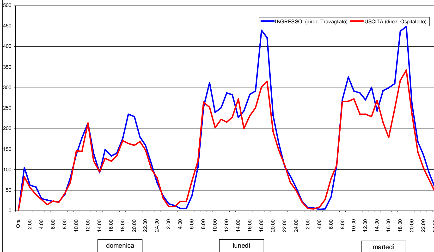
Andamento del traffico da domenica 8 maggio a martedì 10 maggio 2011 [veicoli equivalenti]
